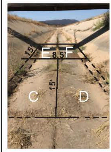
STA 27+85 (C,D,E,F)
