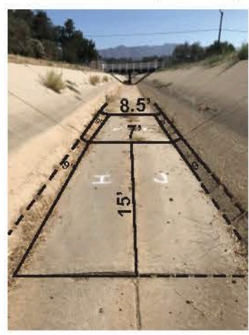
STA 54+30 (I,J,K,L)
